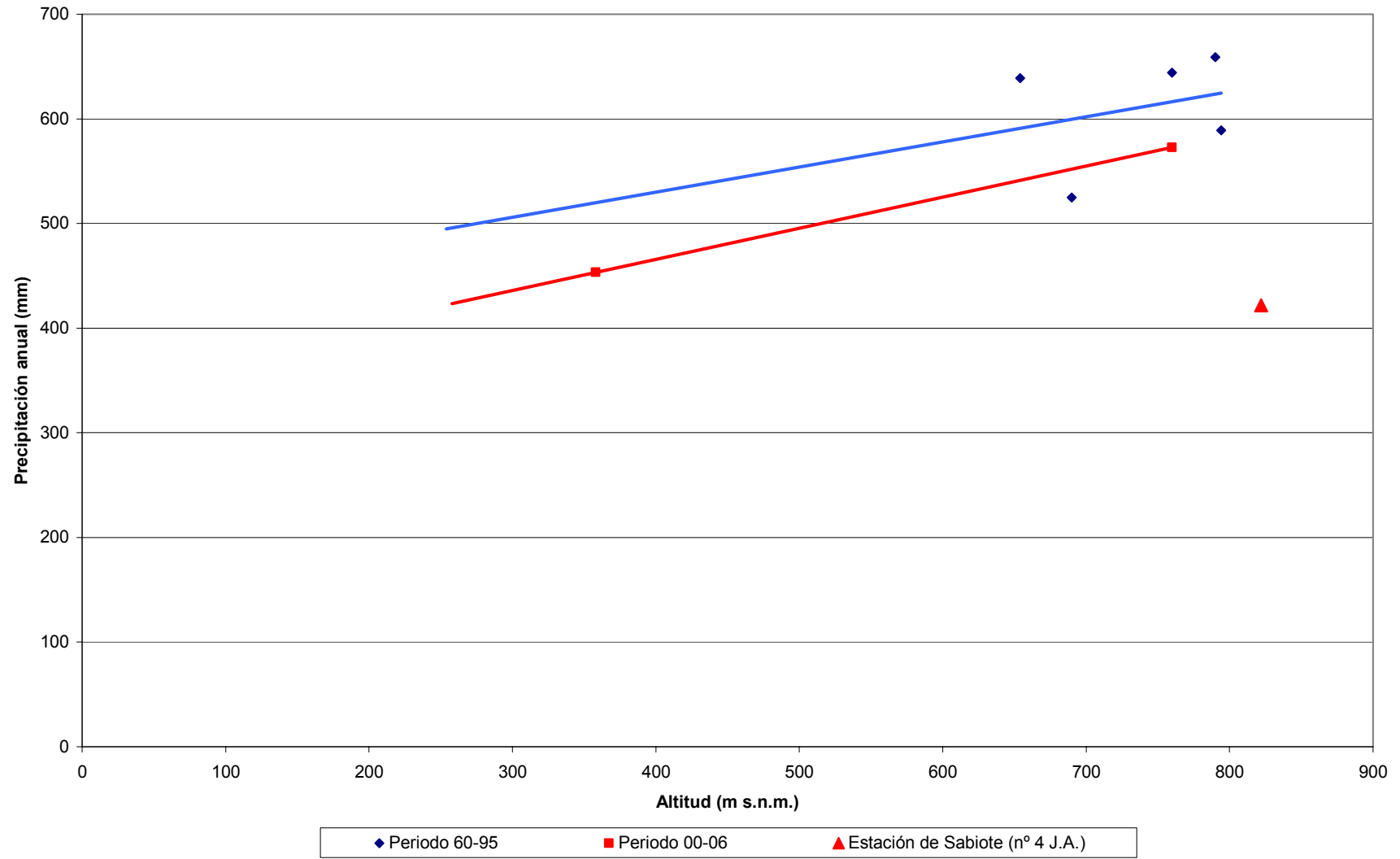
Figura 2.- Relación LLuvia-altitud
