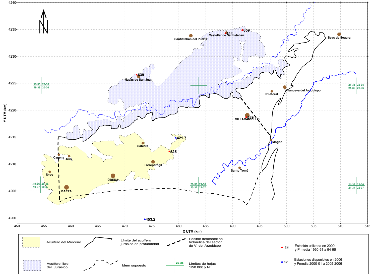
FIGURA 1.- ESQUEMA HIDROGEOLÓGICO DE LA UNIDAD DE ÚBEDA Y ESTACIONES CLIMÁTICAS
